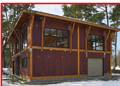
青少年教育施設:野外活動棟／新潟県 H30.3(CLTパネル工法):125m 3 胎内市 2階建て・1棟
